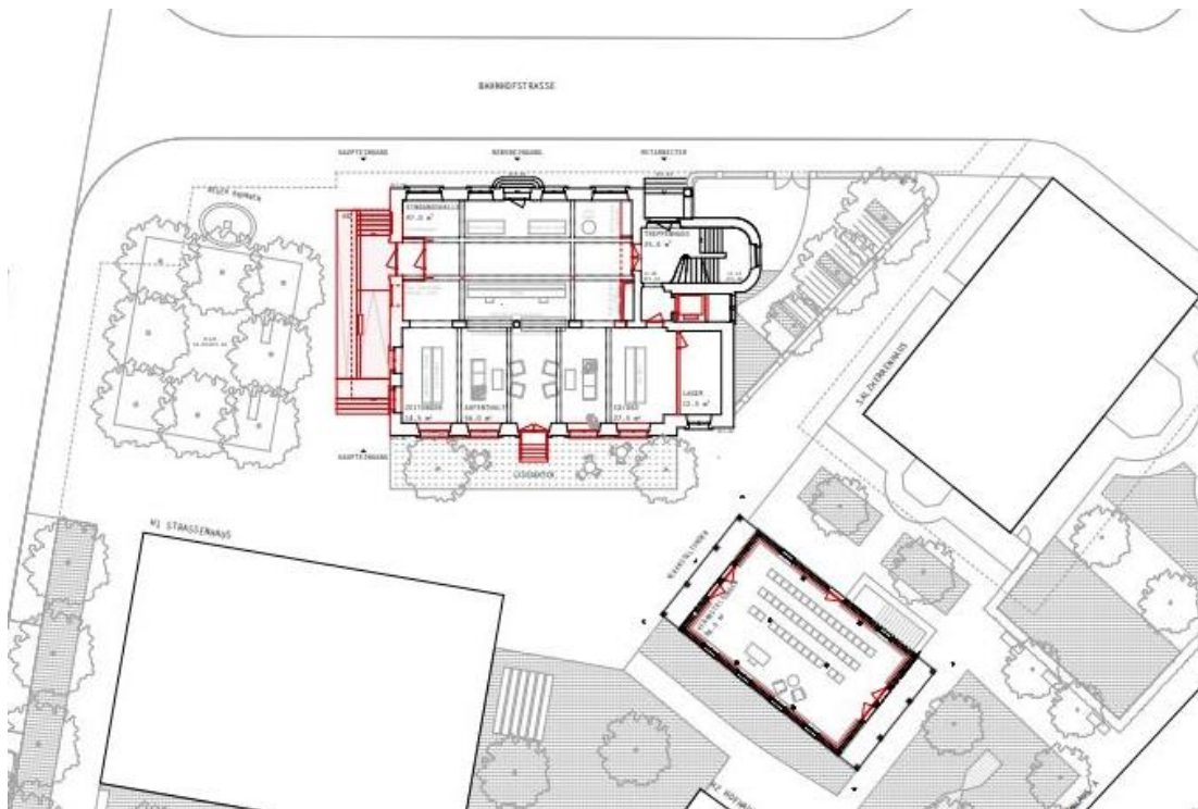
Abb. 3: Grundriss der geplanten Kantonsbibliothek mit westseitigem Haupteingang und Lesegarten im Süden.
