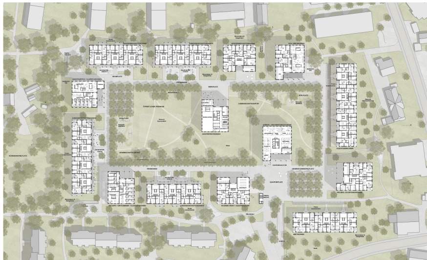
Abb. 9 Situationsplan; «FREIRAUM», ARGE Rykart Architekten AG/Ernst Gerber Architekten + Planer AG mit Klötzli + Friedli Landschaftsarchitekten AG
