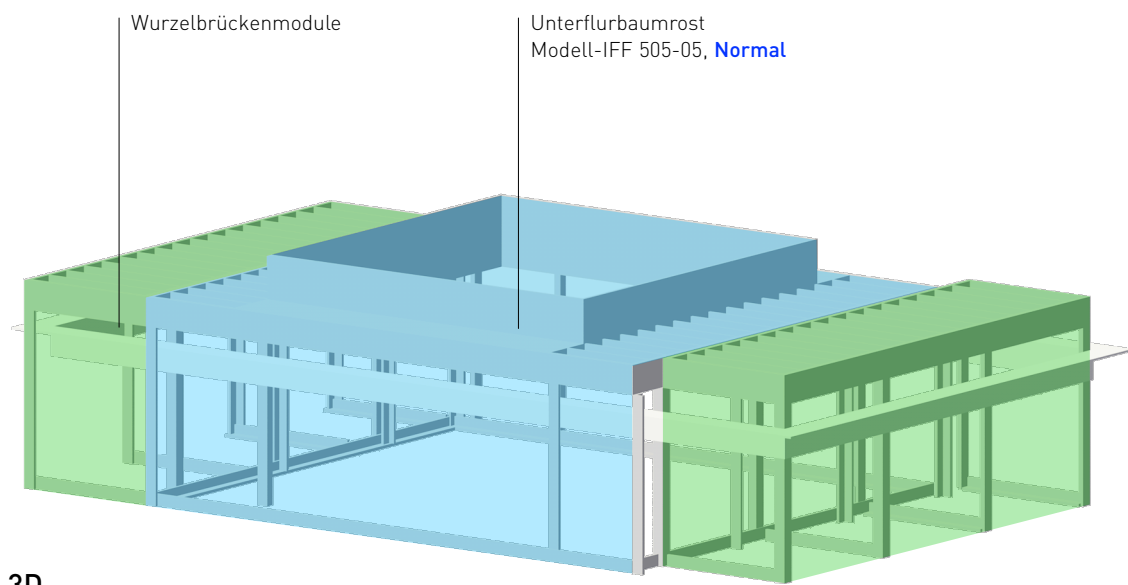
3D Unterflurbaumrost klein
