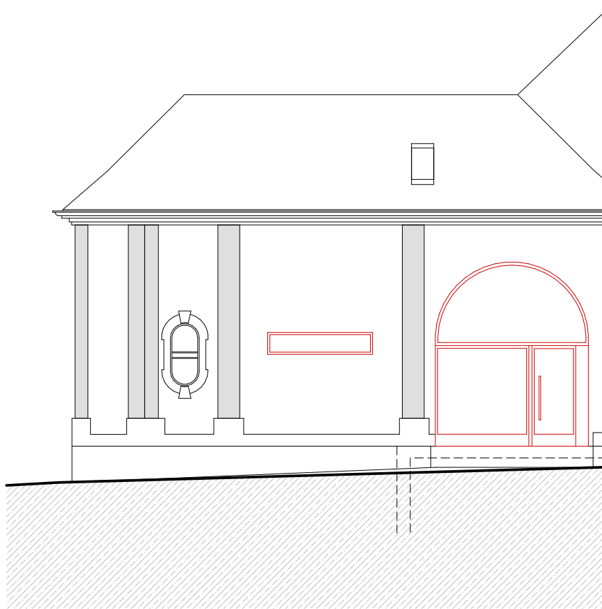
Süd-Fassade
