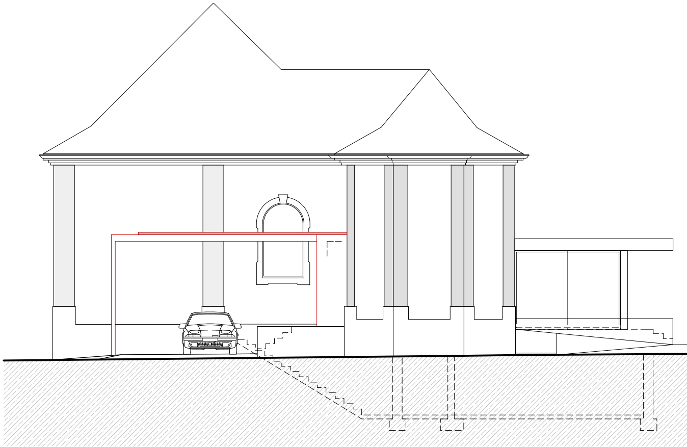
West-Fassade
