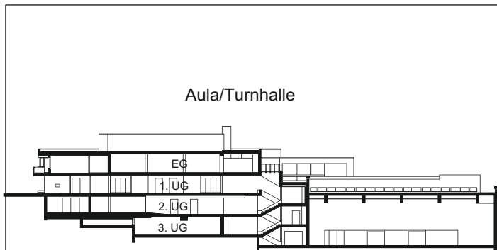
Längsschnitt Bestand
