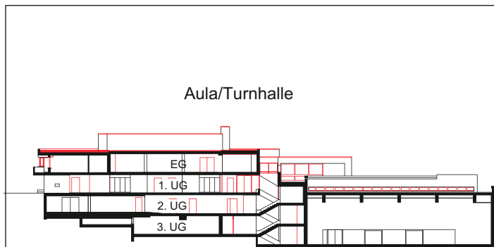
Längsschnitt Projekt
