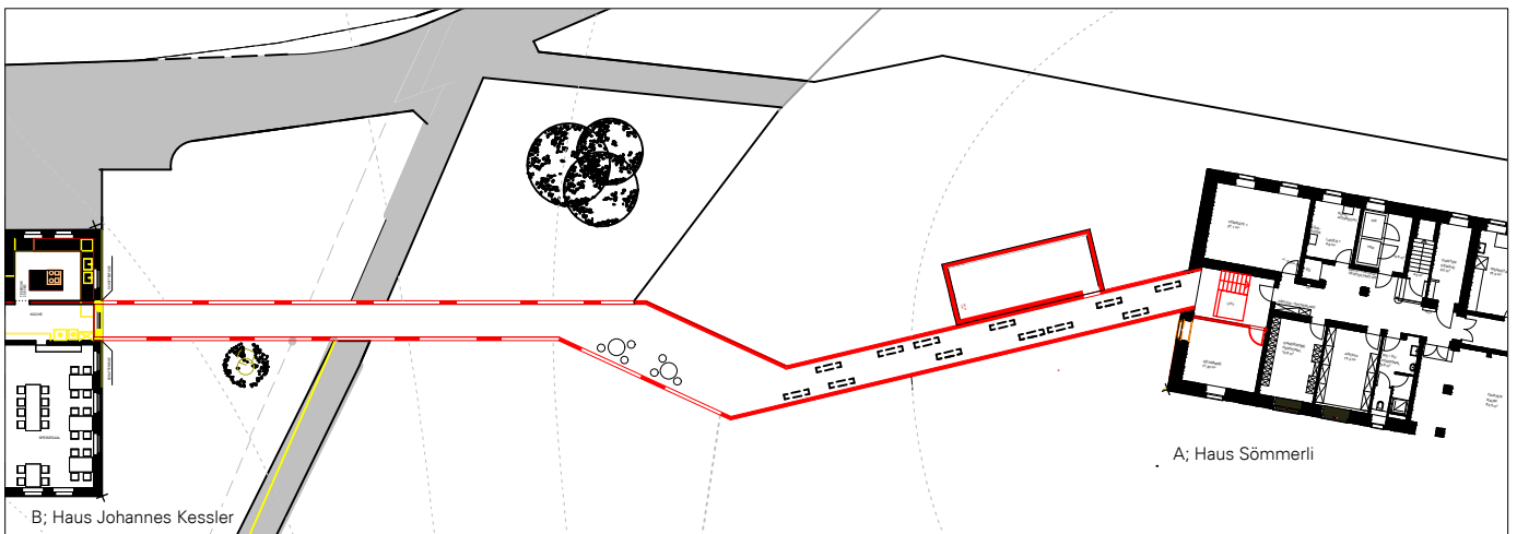
Grundriss Verbindungssteg
