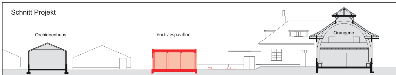
Südostfassade Bestand
